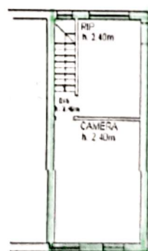
PIANTA PIANO TERZO
